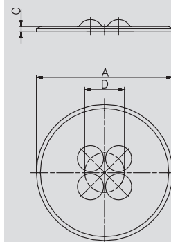
Kontermutter für Kalottenfuß сферическая гайка для сферической ножки
